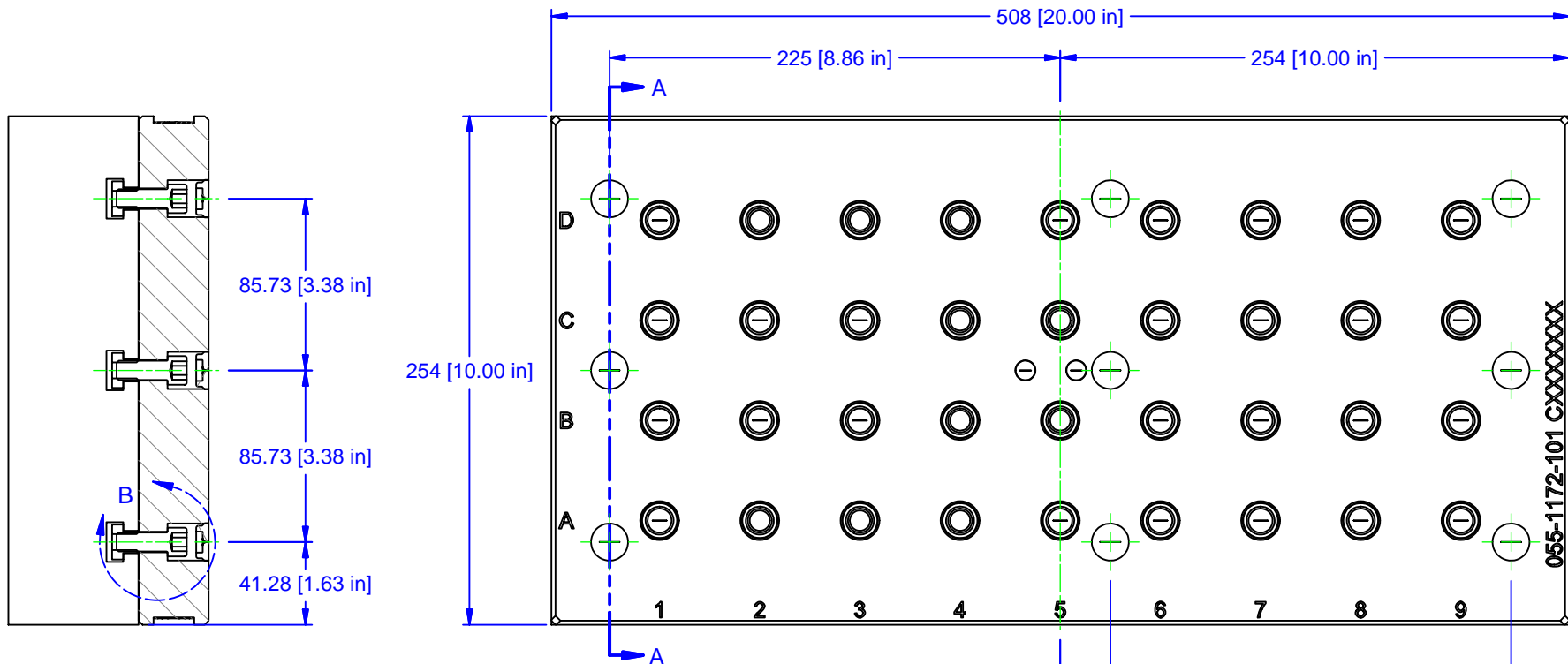
SECTION A-A
